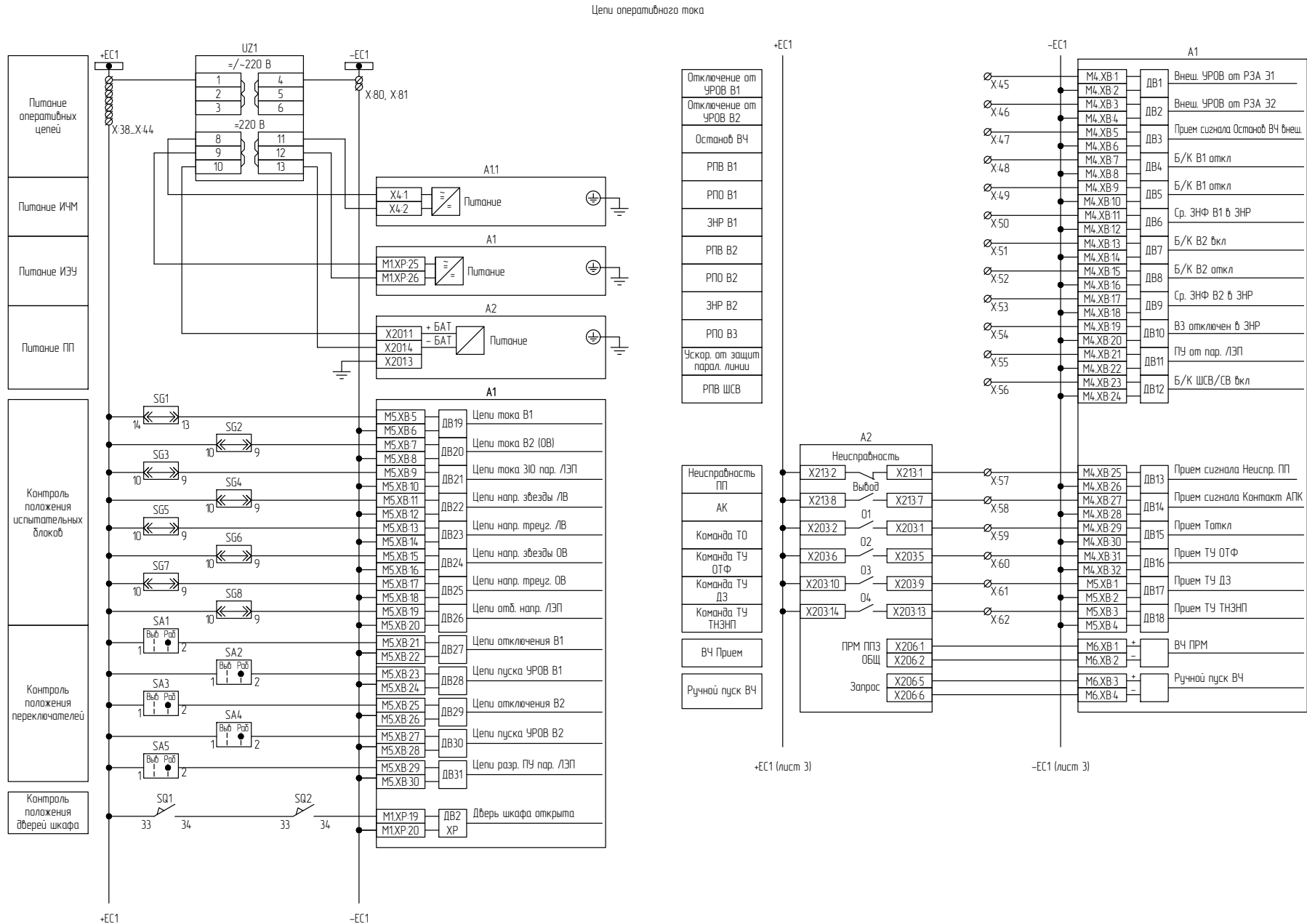
Рисунок В.2 – Схема электрическая принципиальная (часть 2)
